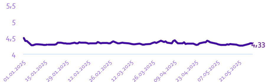
SOFR dinamikasi
